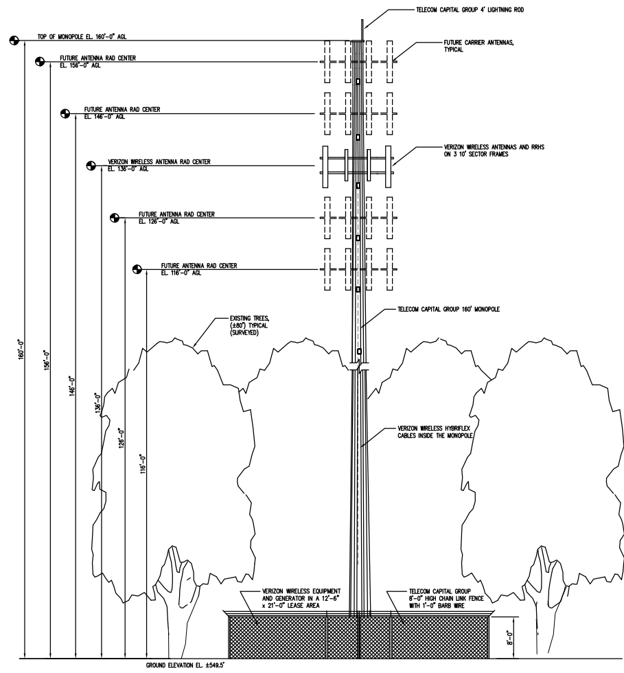
MONOPOLE ELEVATION SCALE: 1/8" = 1'-0"
